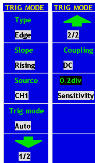
Fig. 33 Edge trigger menu
